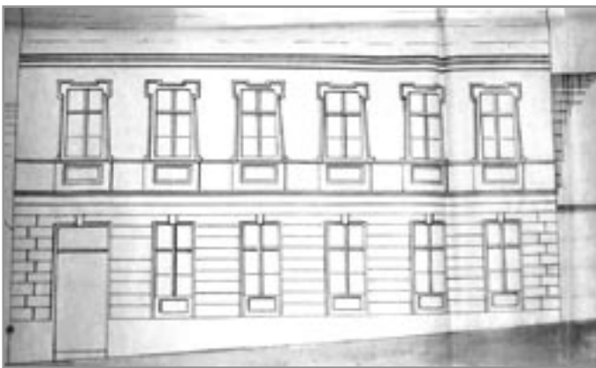
Fotokopie výkresu - Fasáda domu č. p. 6 na Zámecké ulici
