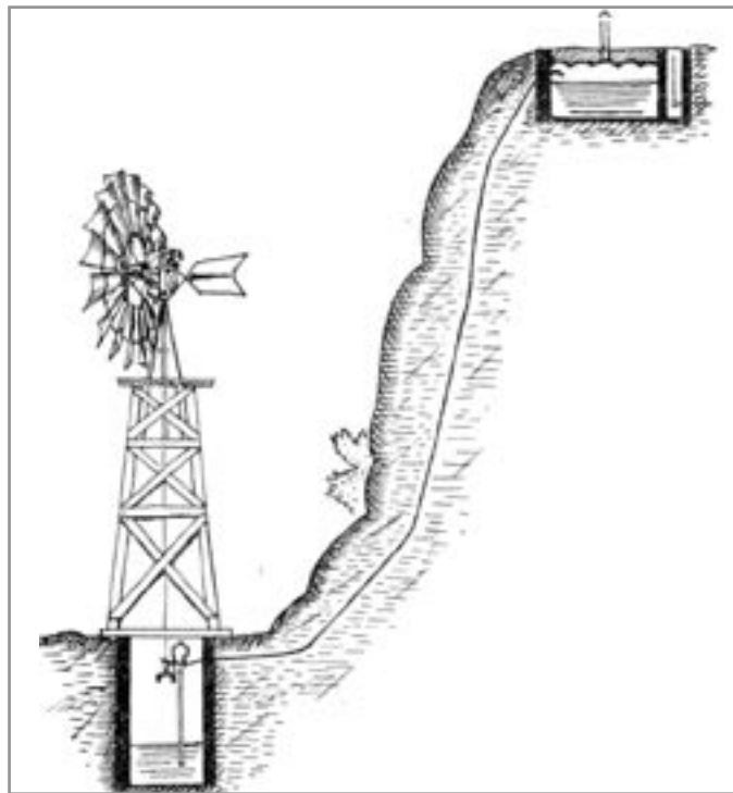
Schema kompletního čerpacího zařízení z dobové školní učebnice (učebnice vlastivědy z roku 1926)
