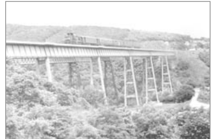
Osobní vlak na novém viaduktu - 20. 6. 1985 foto Jaroslav Valeš
